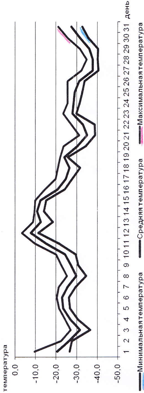
График изменения характеристик температуры воздуха в декабре 1949 г.
